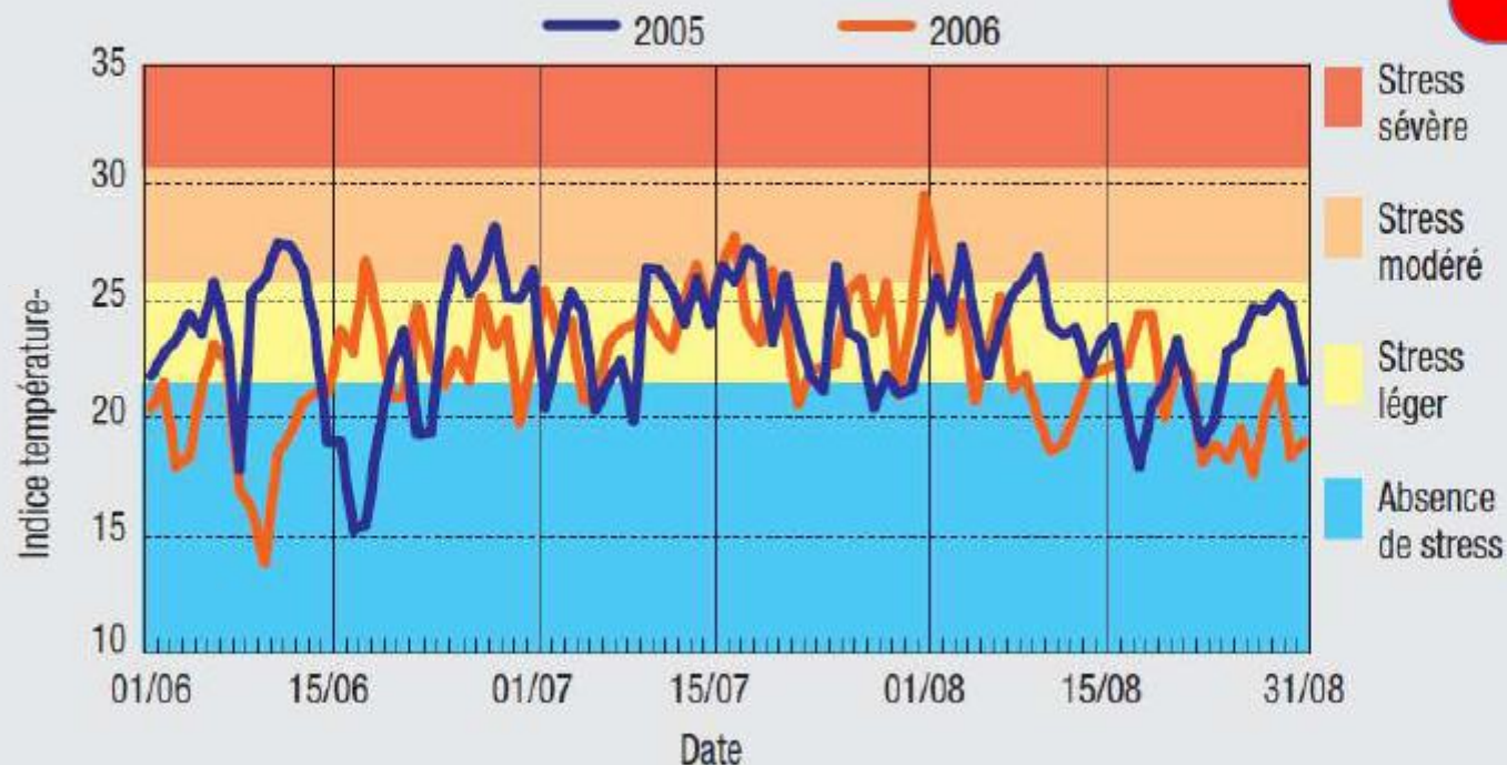
GRAPHIQUE 1 INDICE TEMPÉRATURE-HUMIDITÉ MAXIMAL QUOTIDIEN POUR MONTRÉAL POUR LES ÉTÉS 2005 ET 2006
